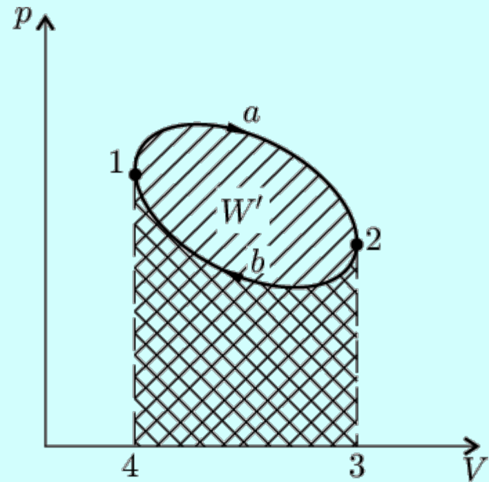
Kruhový děj
