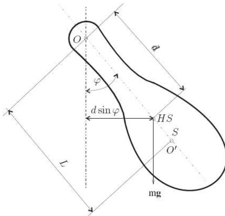
Fig. 1. Reversible pendulum
